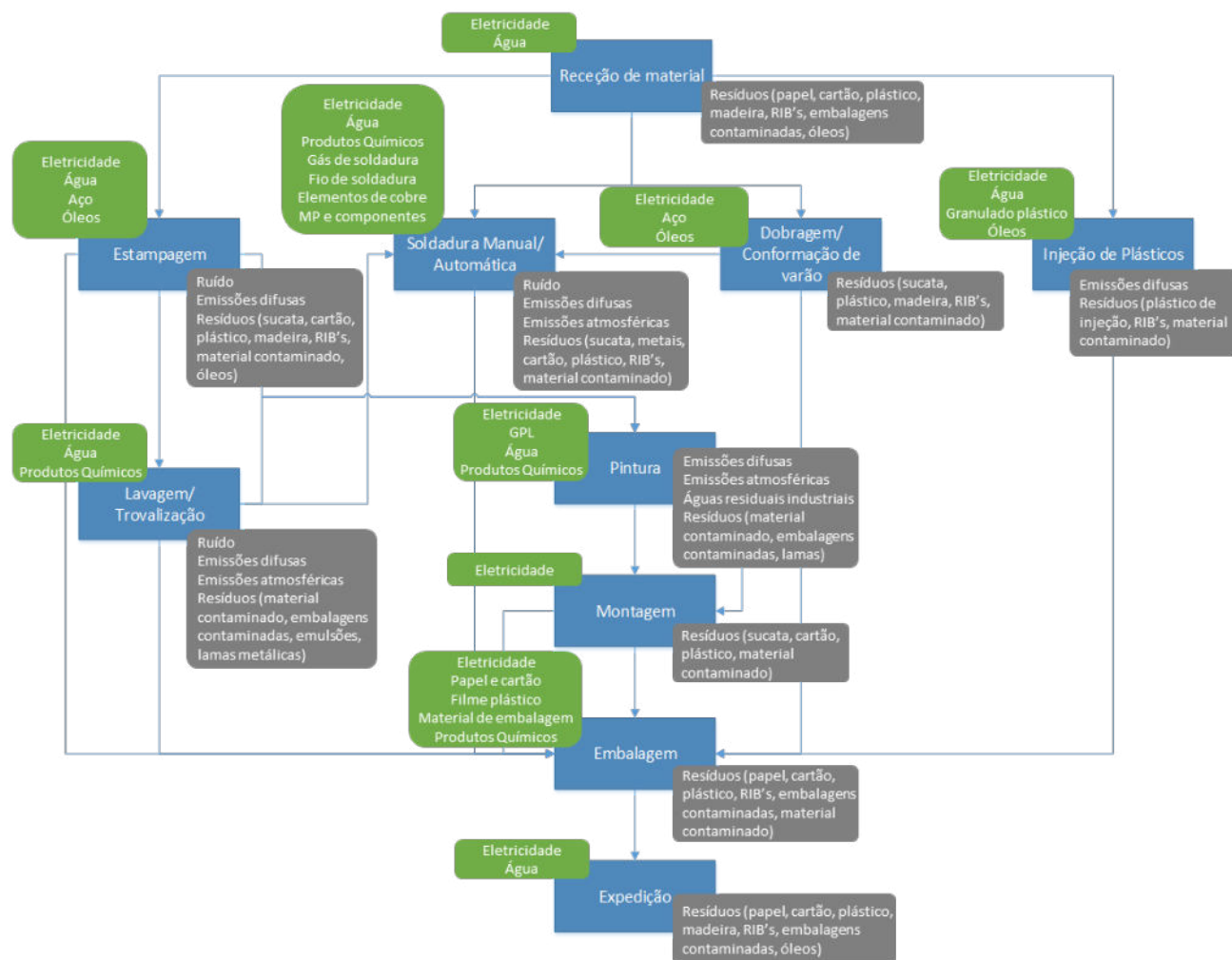
Figura 21 – Esquema representativo dos aspetos e impactes ambientais da Gestamp Vendas Novas nos Processos Produtivos.
