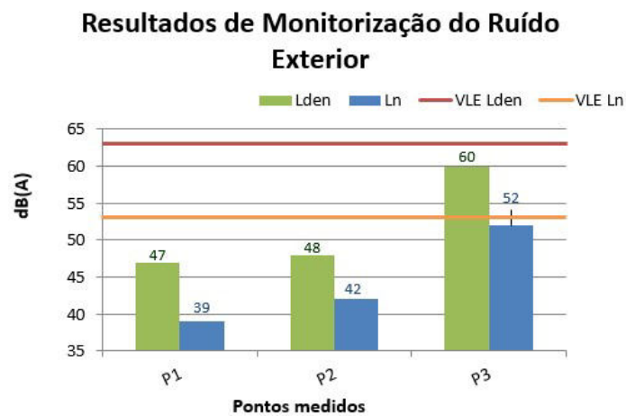
Figura 37 - Representação gráfica dos resultados de monitorização do ruído da fábrica.
