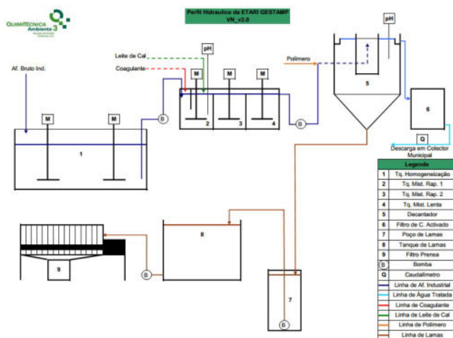
Figura 38 - Diagrama do Sistema de Tratamento da Gestamp VN.
