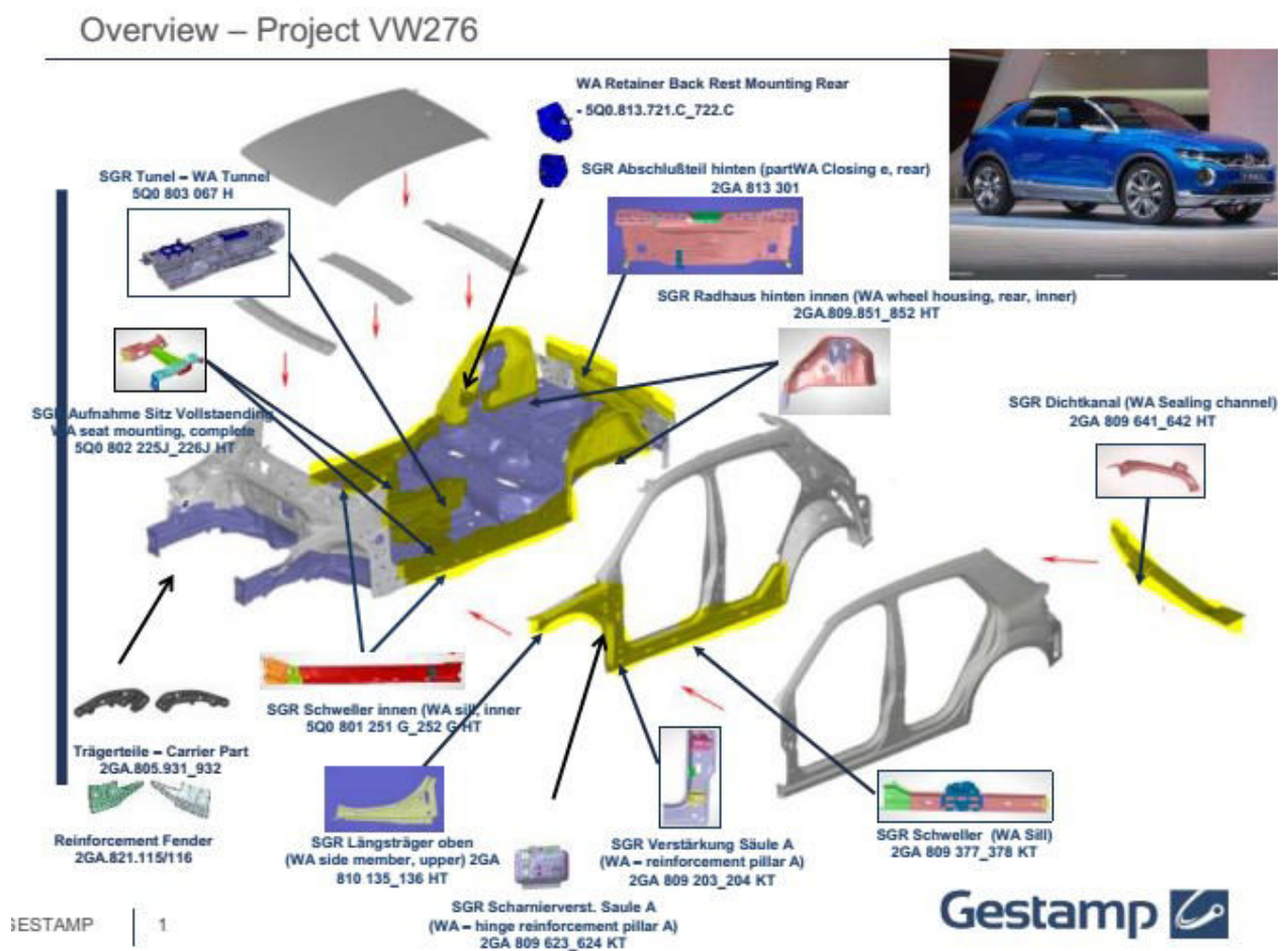
Figura 13 – Produtos do projeto VW 276 – Modelo T-ROC
